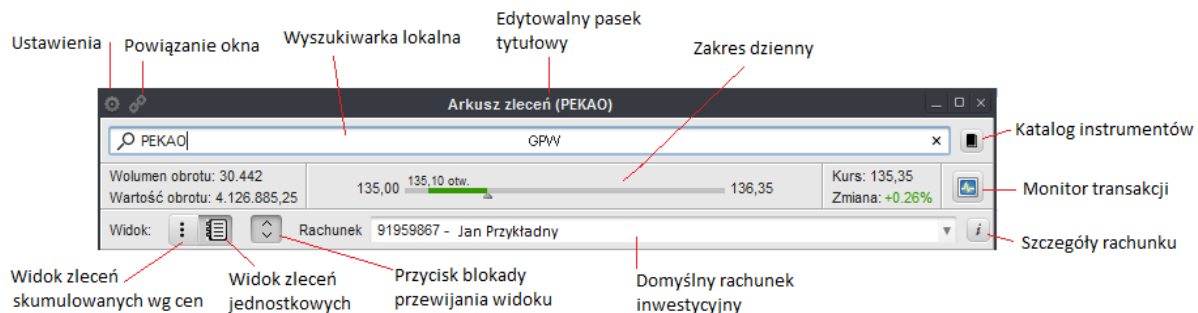
Rys. 2. Widok na pasek zarządzania oknem arkusza zleceń.
